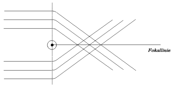
Abbildung IV.2: Gravitationslinse
