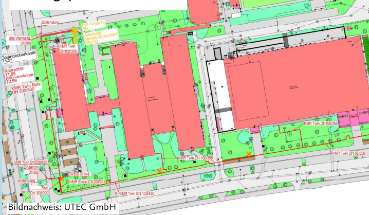
Leitungsplan - Ausschnitt
